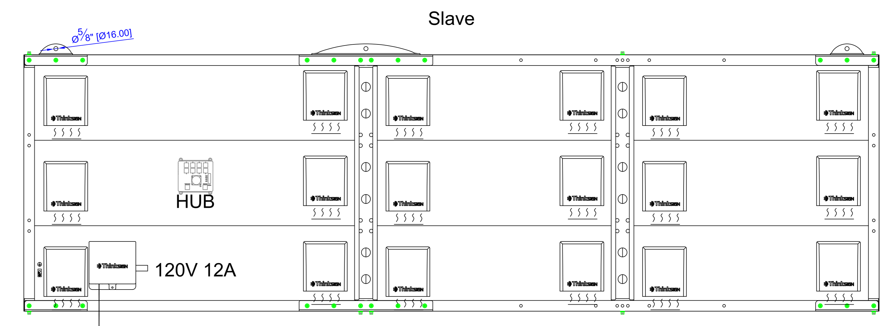
NET CABLE 5E
